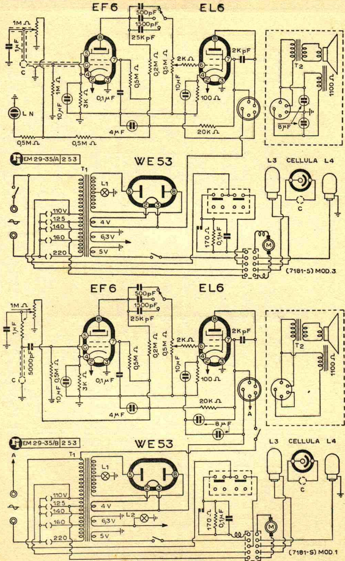
Amplificatori PEM I (sopra) e PEM III (sotto) per cine sonoro 16 mm.
